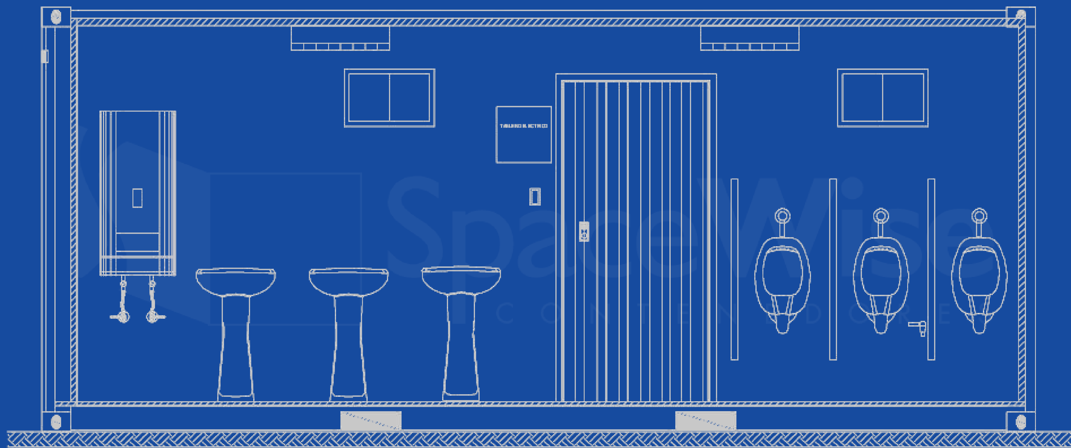
CORTE A-A
